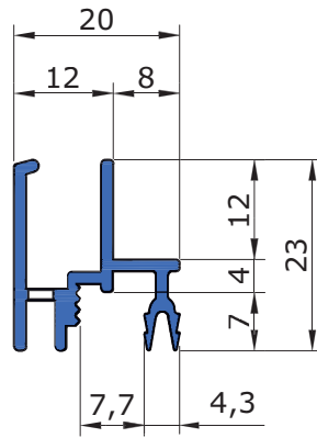
AL 0300 con terminali
