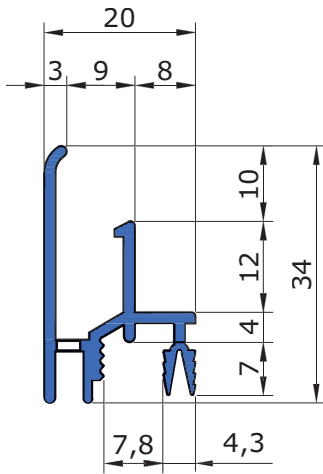
AL 0320 con terminali LOTTO MINIMO 1500 m
