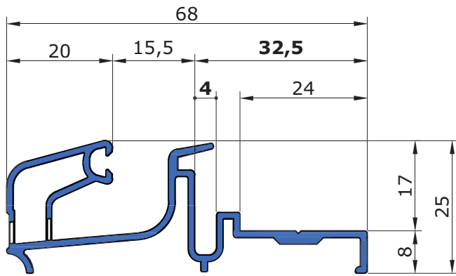
AL 3700 INTERCAMBIABILE CON AT 8590
