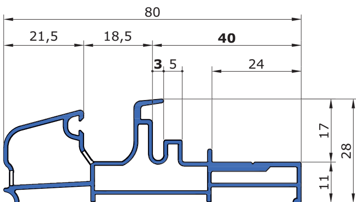
AL 3990 INTERCAMBIABILE CON AT 8930 LOTTO MINIMO 650 m
