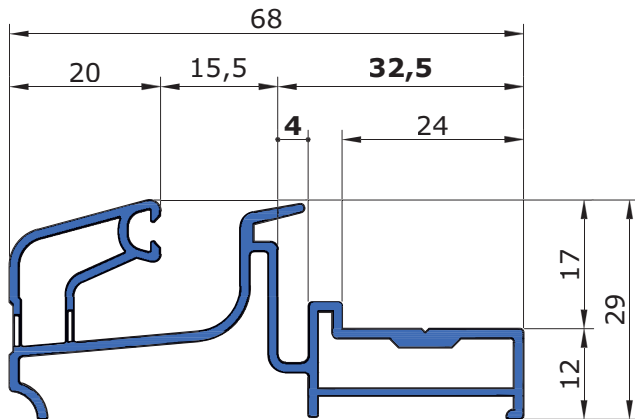
AL 3710 INTERCAMBIABILE CON AT 8600
