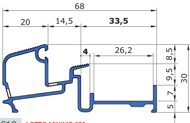
AL 3810 LOTTO MINIMO 850 m
